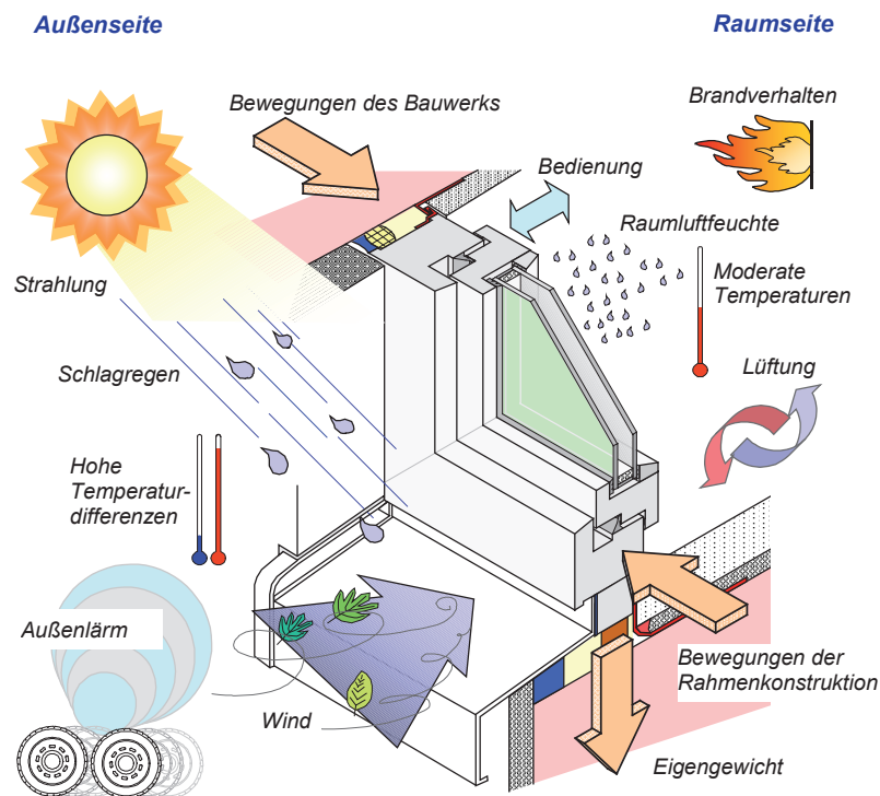
Schematische Darstellung von Einwirkungen auf den Anschluss von Fenstern
