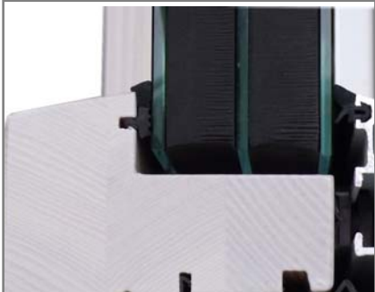
Trockenverglasung (innen und außen) / Glasleistenkontur - schräg
