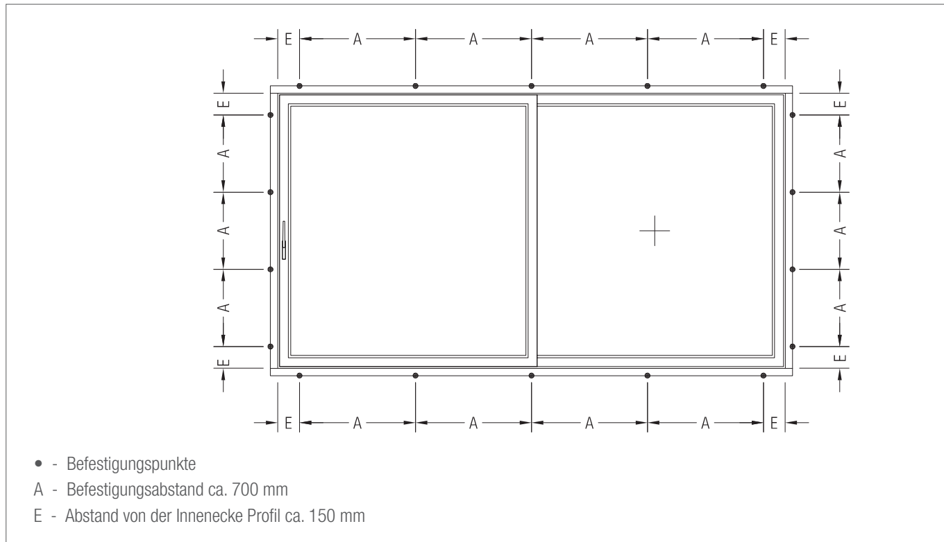
Abb. 2: Befestigungsabstände für Hebepanorama
